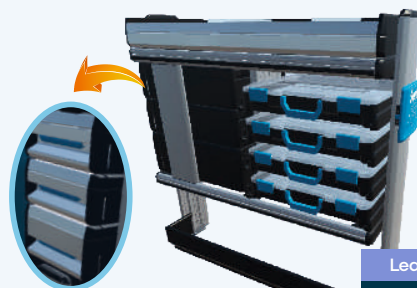
Højre SR5 SMH6 1018x356x969 mm. [BxDxH] Vægt: 56 kg. [FL-SMH6]
